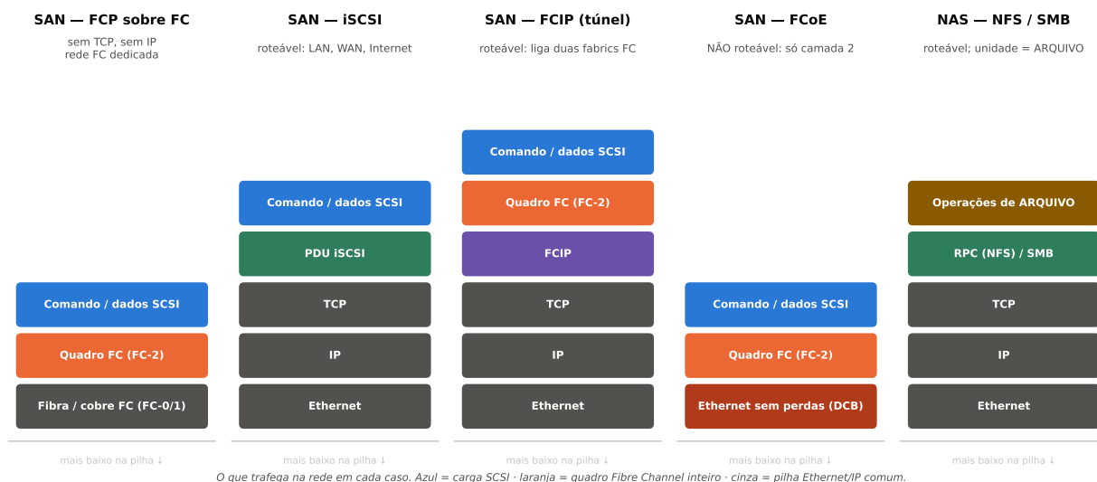
Figura 2: O que trafega na rede em cada arquitetura. Três leituras que a figura torna imediatas: (i) iSCSI e FCoE não são variantes um do outro — o iSCSI carrega comandos SCSI sobre TCP/IP, enquanto o FCoE carrega o quadro FC inteiro sobre Ethernet; (ii) FCIP e FCoE carregam a mesma coisa (o quadro FC), e diferem apenas em sobre o quê — daí um ser roteável e o outro não; (iii) o NAS é o único em que a unidade não é o bloco : no topo da pilha há operações de arquivo, e não comandos SCSI. Essa última diferença é a da Seção 3, e é a que decide tudo o mais.
